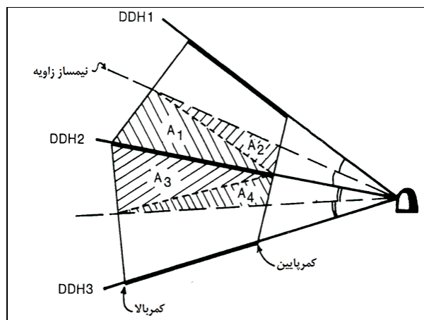
شکل ۴-۱۶- تعیین عیار متوسط پهنه‌های استخراجی به کمک چال‌های بادبزنی (A: بلوک‌های اکتشافی تکمیلی، DDH: چال)
