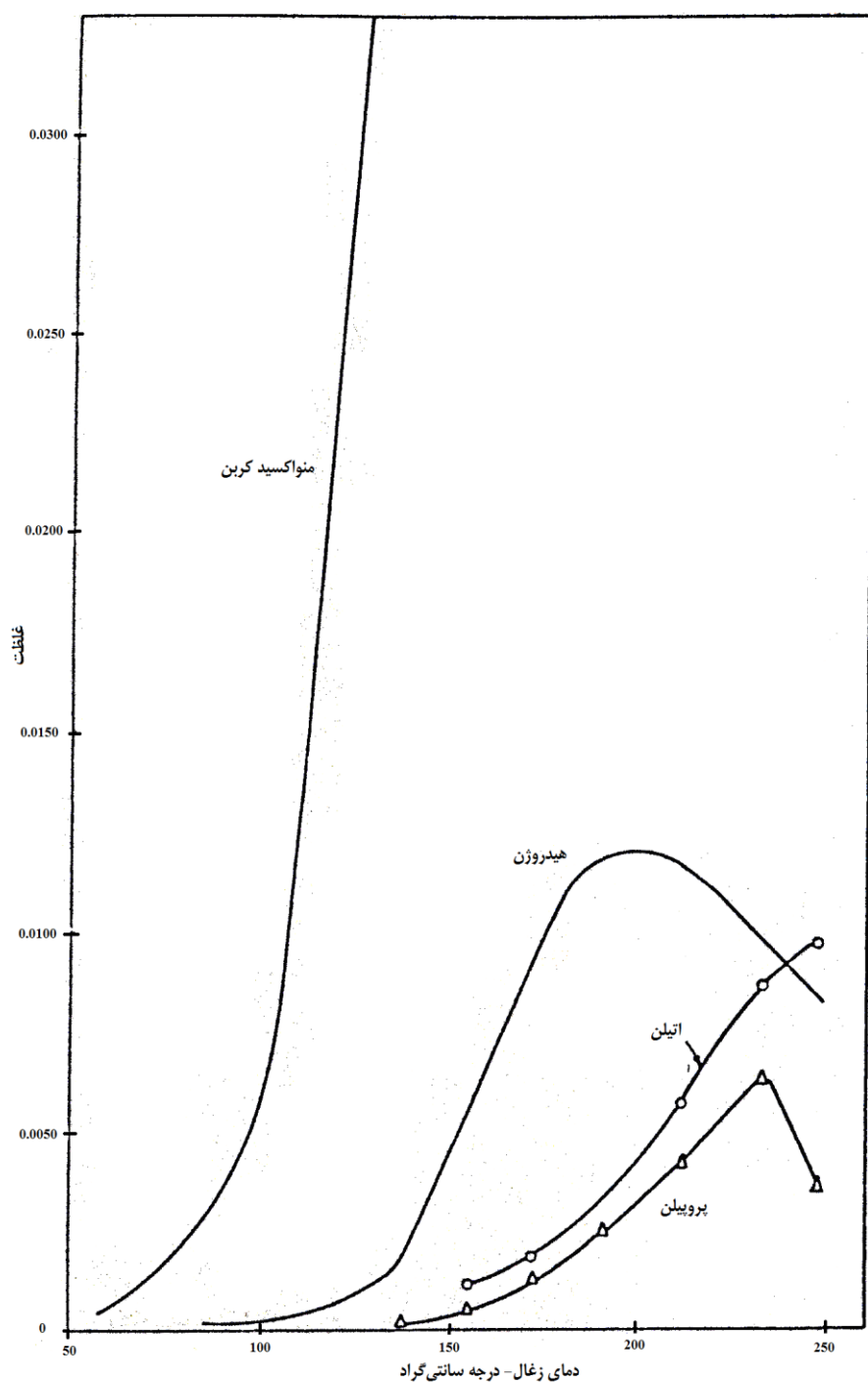
شکل ۷-۱- یک منحنی نمونه‌وار آزمایش اکسایش زغال
