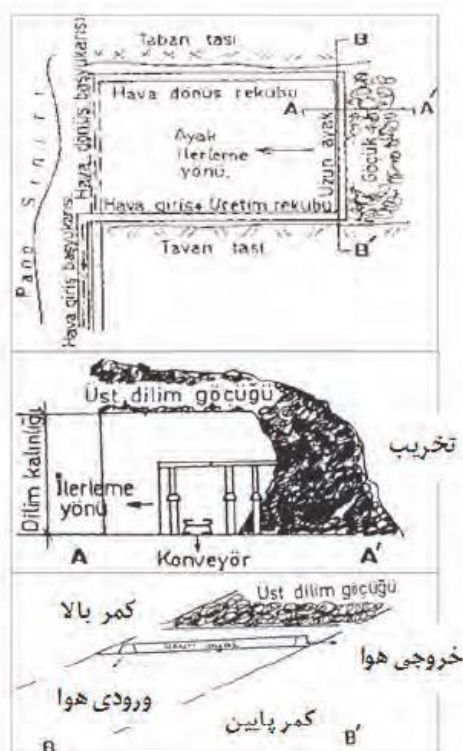
شکل پ ۳-۵- روش استخراج لایه‌های ضخیم در منطقه
