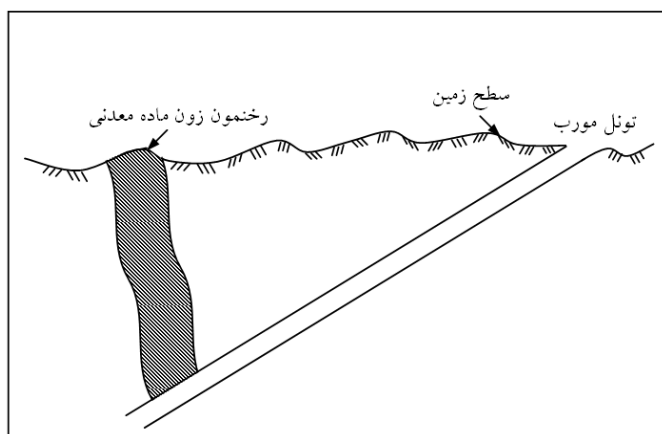
شکل ۱-۲- تونل مورب
