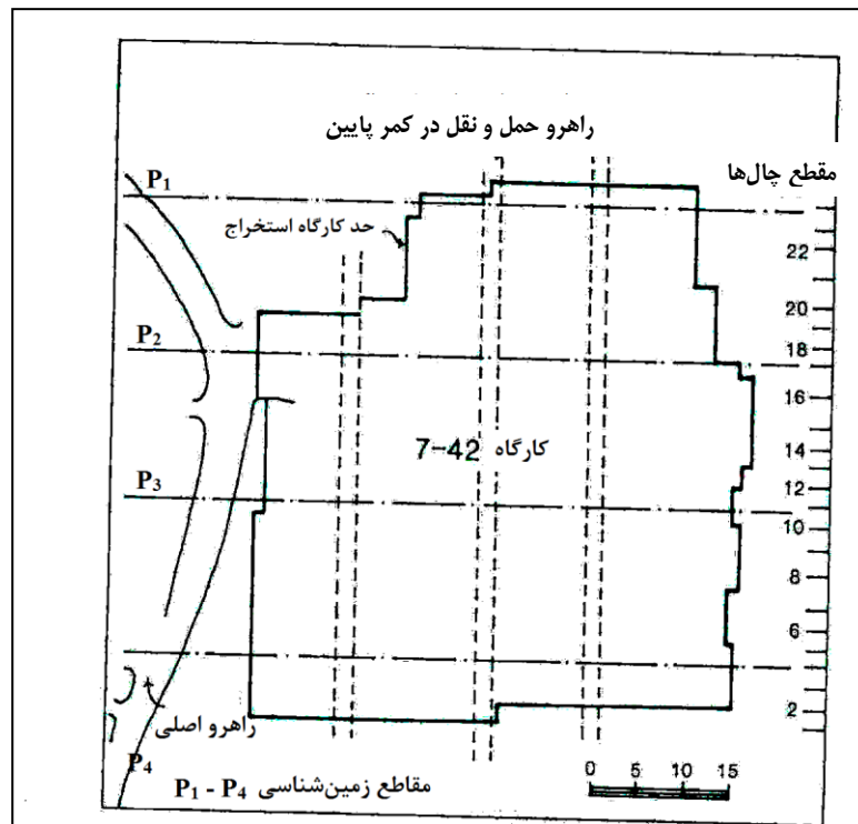
شکل ۴-۱۸- نقشه یکی از کارگاه‌های استخراجی شکل ۴-۱۷
