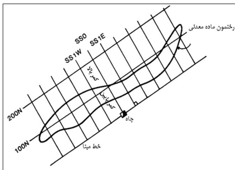
شکل ۵-۱-۱-۱- جانمایی مقاطع معدنی در محدوده کانسار
