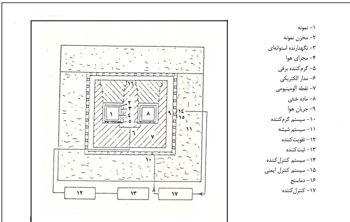
شکل ۷-۳- کالریمتر تک دمای مدل کالوت
