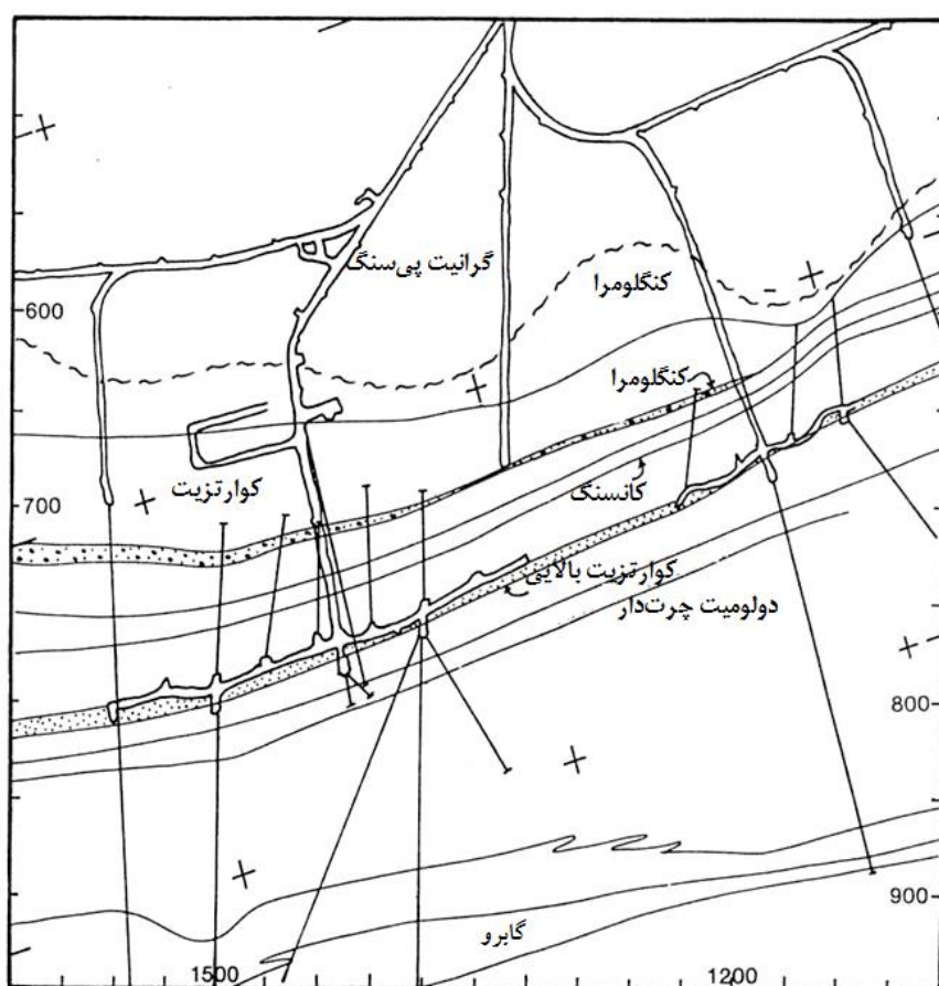
شکل ۱-۱۰- نمونه‌ای از نقشه طبقات معدن در یکی از معادن مس زامبیا
