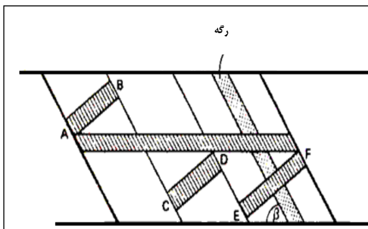
شکل ۳-۱۴- نمونه برداری شیاری تفکیکی از دیواره یک تونل دنبال رو (AB, CD, EF نمونه های جزئی و AF مغزه کلی است.)
