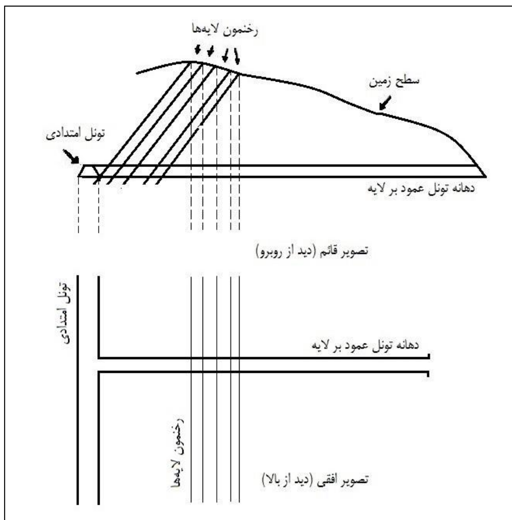
شکل ۲-۷- تونل امتدادی
