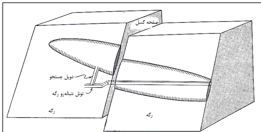
شکل ۵-۷- حفر دویل برای یافتن بخش قطع شده ماده معدنی به وسیله یک گسل پرشیب
