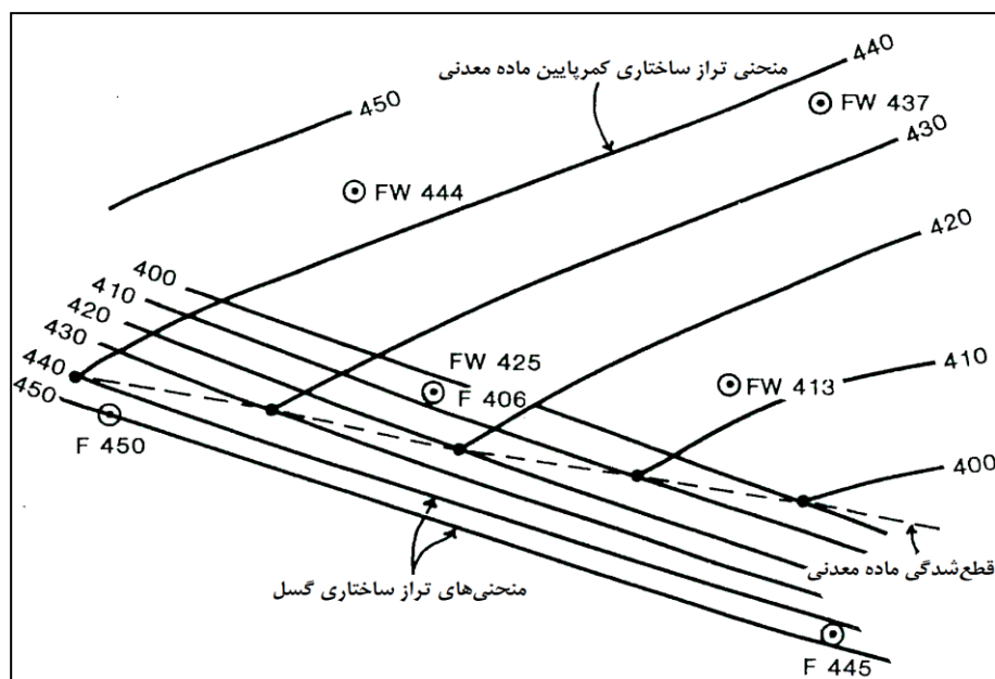
شکل ۴-۹- منحنی‌های تراز ساختاری کمرپایین یک توده معدنی همراه با منحنی‌های گسلی که آن را قطع کرده است.
