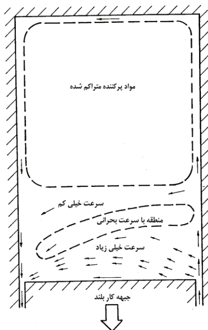
شکل ۷-۶- جبهه کار استخراج پسرو و نشت هوا
