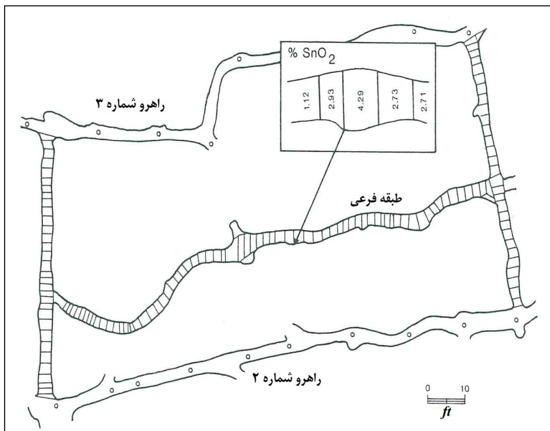
شکل ۴-۲- نمونه‌ای از نقشه‌های مایل که در آن موقعیت طبقات فرعی و دیول‌ها به نمایش درآمده است.
