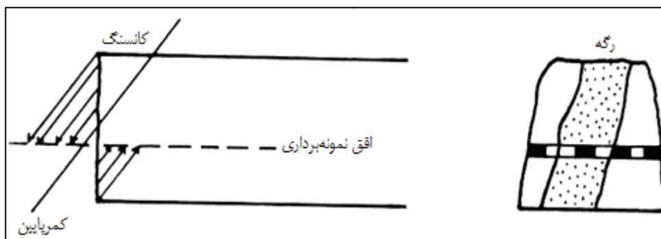
شکل ۳-۷- نمونه‌برداری از جبهه‌کار تونل دنباله‌رو
