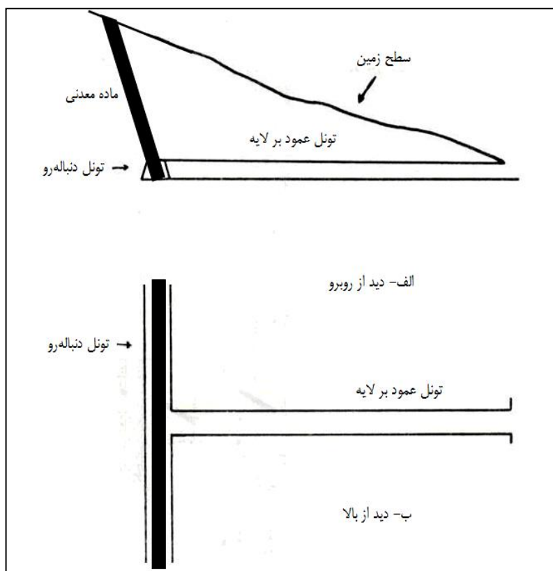
شکل ۲-۱۳- تونل دنباله‌رو
