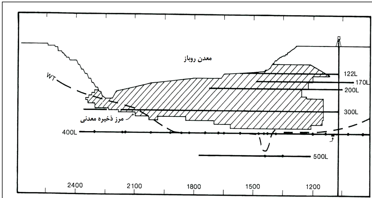
شکل ۳-۴- نقشه تصویر شده در سطح قائم که نشانگر افق‌های معدن روباز و محدوده ماده معدنی است.
