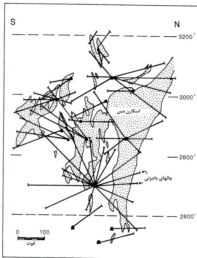
شکل ۴-۱۵- چال‌های اکتشافی بادبزنی در یک معدن مس اسکارنی
