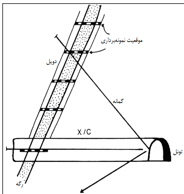
شکل ۳-۱۱- نمونه برداری در تونل‌های امتدادی
