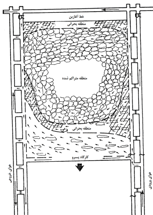
شکل ۷-۸- مناطقی در کارگاه پسرور که بیشترین احتمال خودسوزی را دارند.
