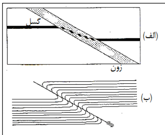
شکل ۵-۹- تشخیص گسل در حفاریات استخراجی با مشاهده کشیدگی طبقات الف- کشیدگی و شکستگی ماده معدنی ب- کشیدگی و کج شدن طبقات در مجاورت گسل
