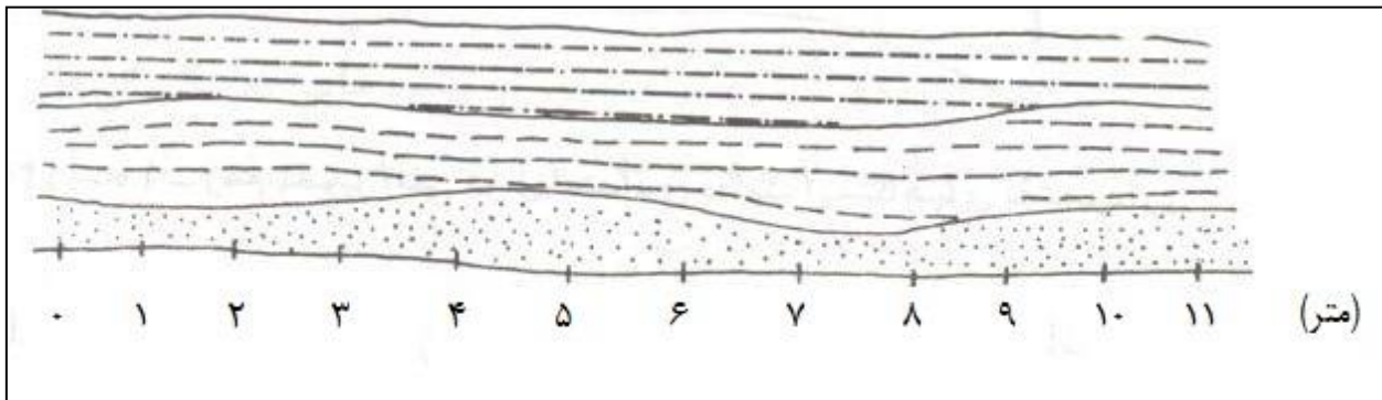
شکل ۲-۱۱- تصویر تکمیل شده سقف تونل امتدادی
