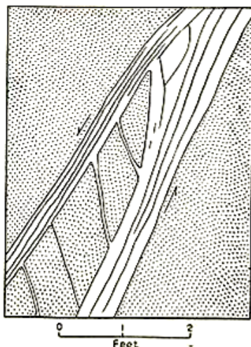
شکل ۵-۱۱- شکستگی‌های برشی در سنگ‌های اطراف گسل
