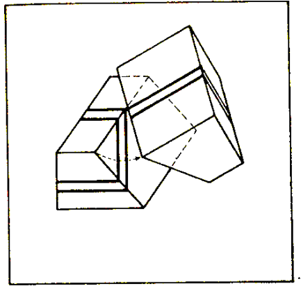
شکل ۵-۲- گسل با حرکت چرخشی
