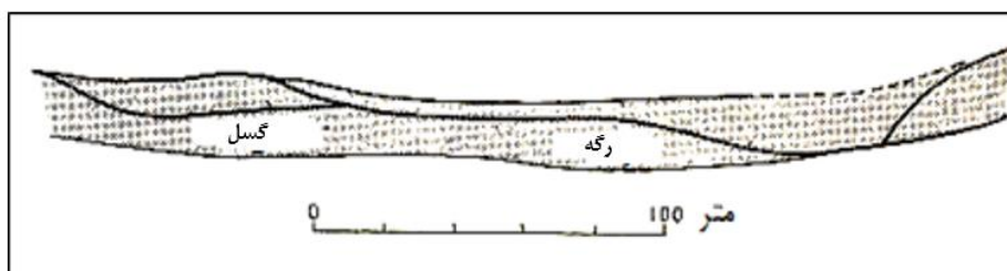
شکل ۵-۱۲- تشخیص اشتباه سطح گسل با دیواره رگه
