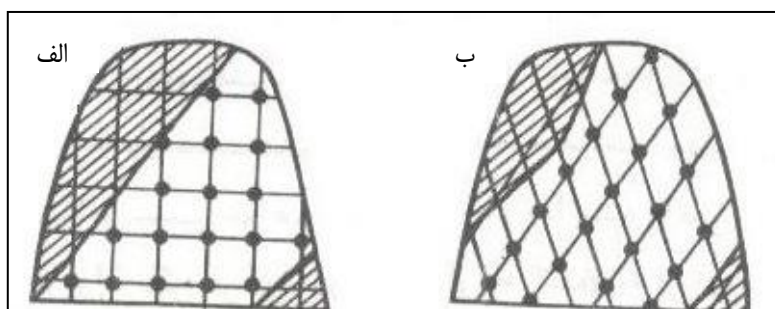
شکل ۳-۱۶- نمونه‌برداری نقطه‌ای در جبهه کار تونل‌های دنباله‌رو
