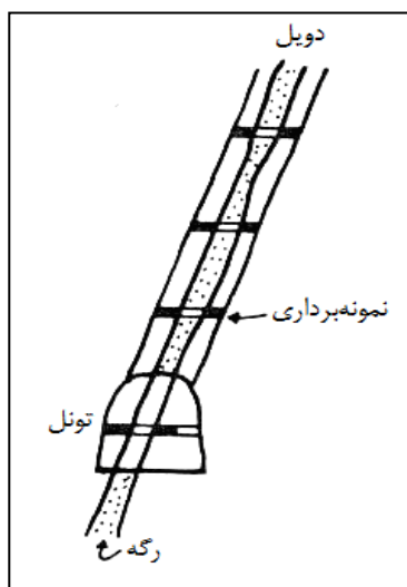
شکل ۳-۱۰- موقعیت نمونه برداری در دویل
