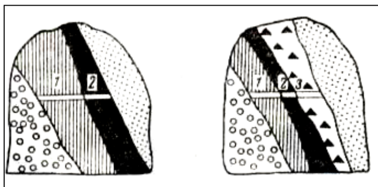
شکل ۳-۱۵- نمونه برداری شیاری تفکیکی
