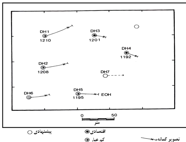
شکل ۱-۹- نقشه حفريات اکتشافی
