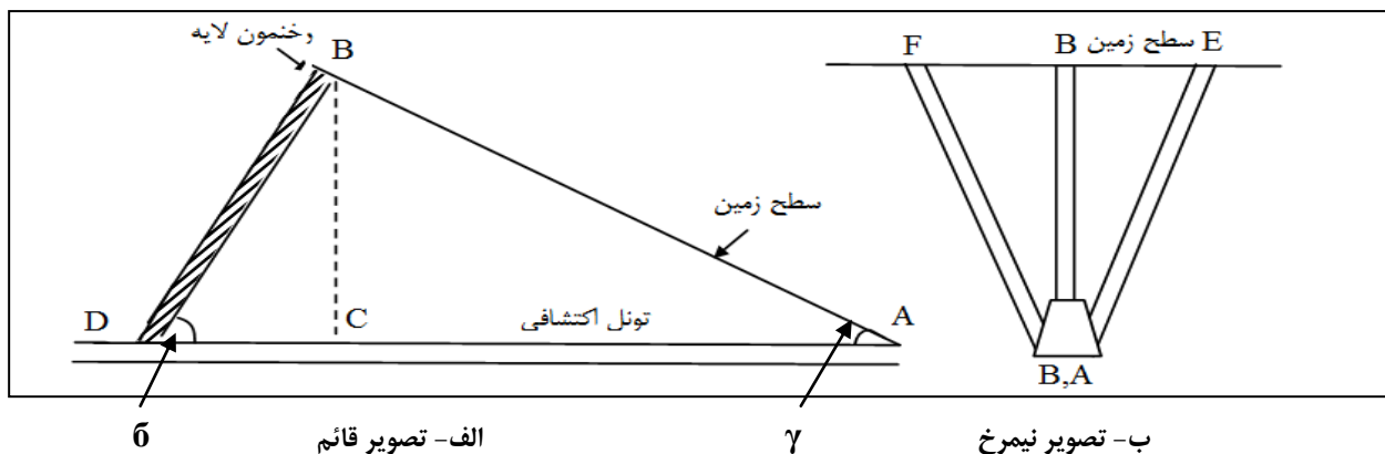
شکل ۲-۱۷- وضعیت‌های مختلف حفر دویل
