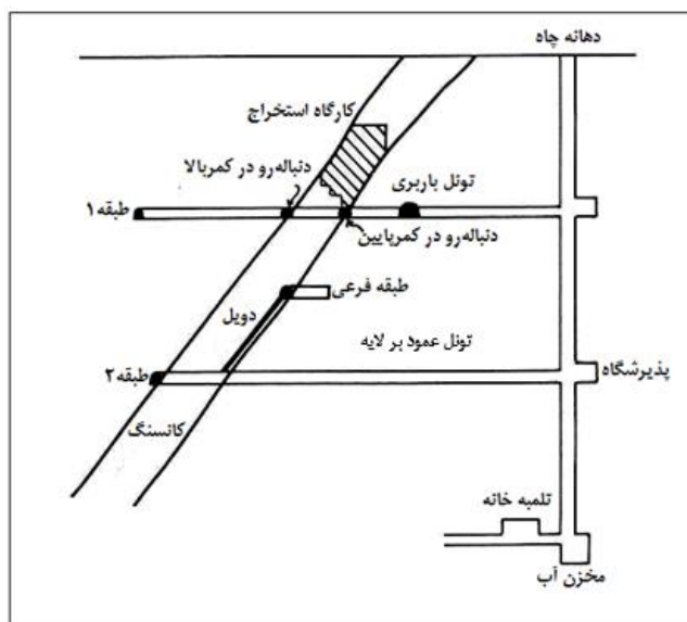
شکل ۳-۱- چاه و سایر حفاریات استخراجی
