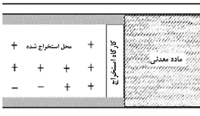
شکل ۱-۴-۱- کارگاه استخراج
