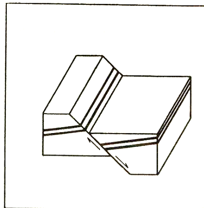
شکل ۵-۴- گسل شیب لغز
