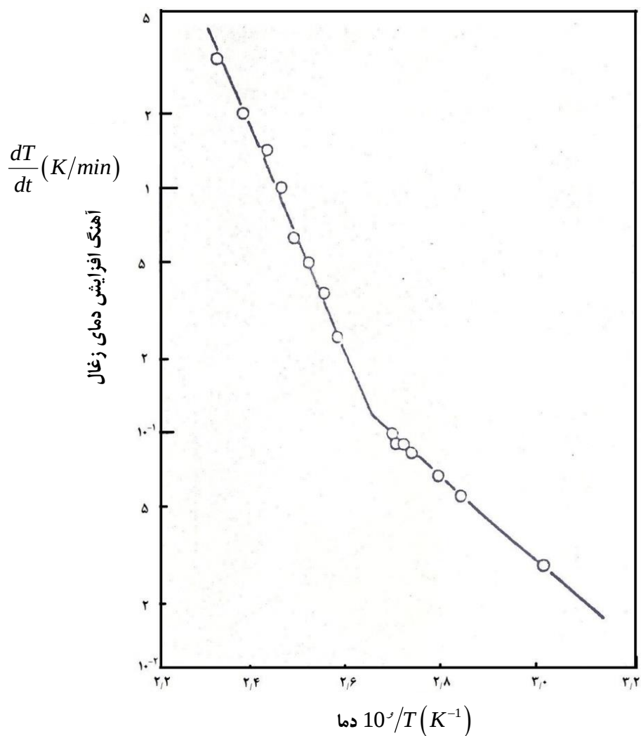
شکل ۷-۲- نمونه‌واری از منحنی‌های آرنیوس
